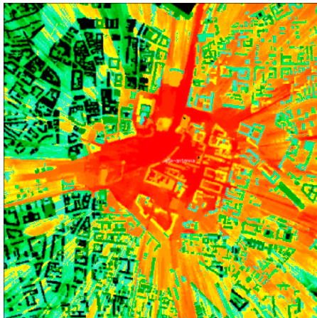
Abb. 3: Prädiktion der Signalstärke einer GSM-Antenne
