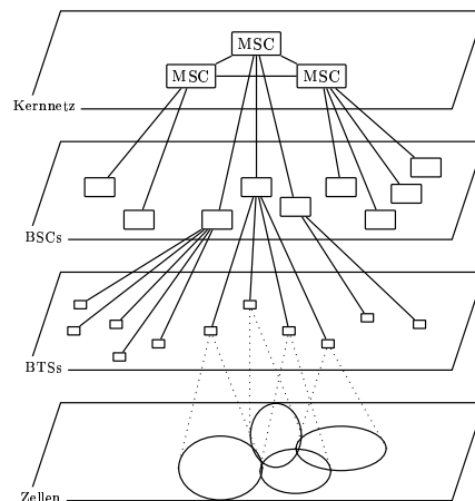
Abb. 1: Hierarchische GSM-Infrastruktur
