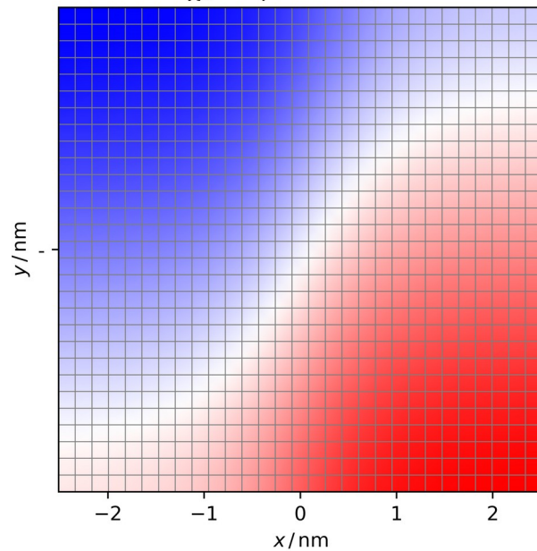
\chi_1 - SqRA + PCCA+
