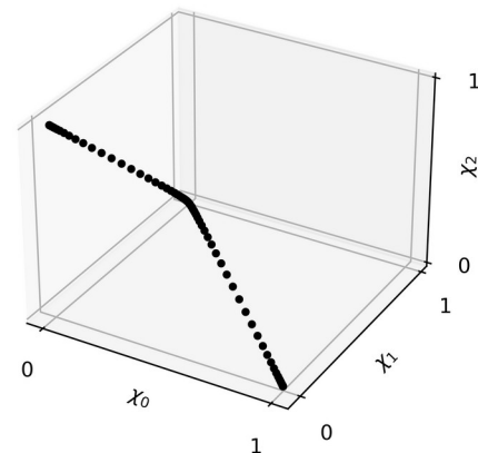
2-simplex \chi_0, \chi_1, \chi_2
